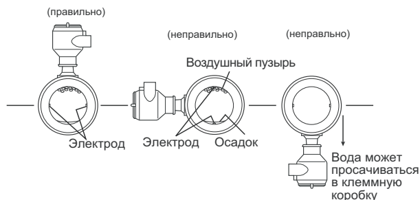
Монтажная ориентация
