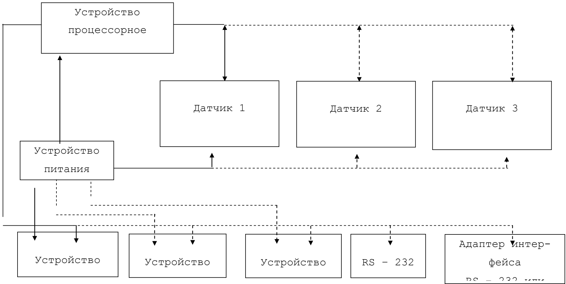
Рисунок 1.2 - Газоанализатор ГАММА-100. Структурная схема газоанализатора с тремя каналами измерения
