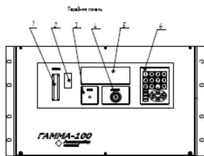
а) газоанализатор GAMMA-100 | три интерфейсных канала
