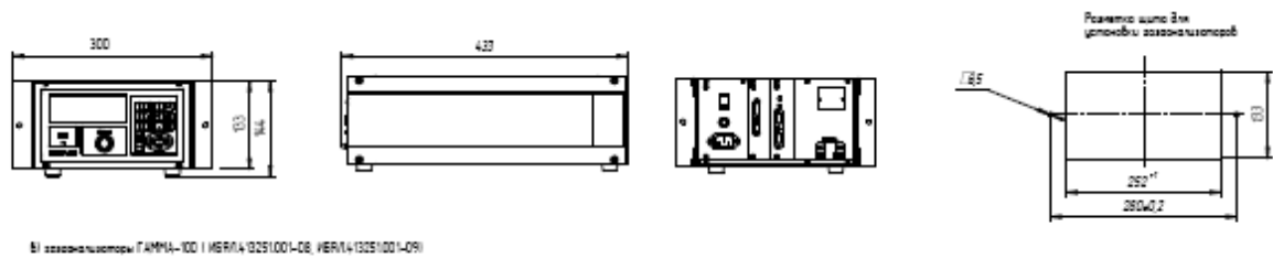
Рисунок 2.1 – Газоанализаторы GAMMA-100. Размеры шлюза для установки газопроанализаторов
