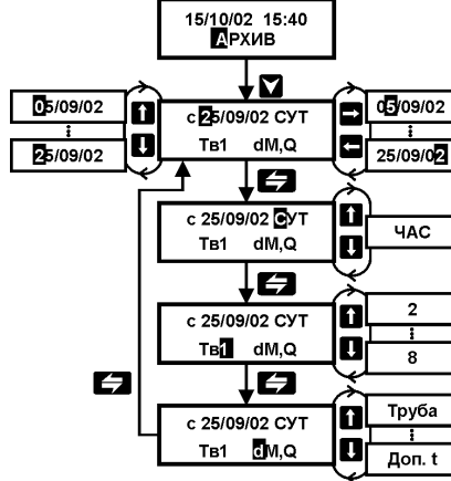
Рисунок 19 – Последовательность действий по просмотру архивной информации
