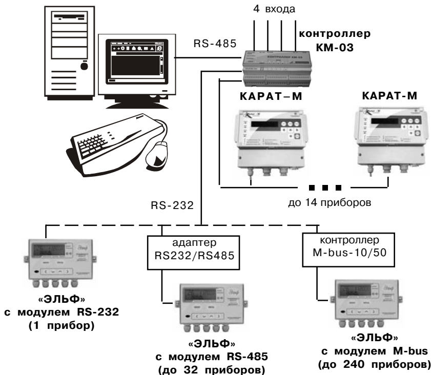
Рисунок 2.3 - Варианты использование контроллера КМ-03
