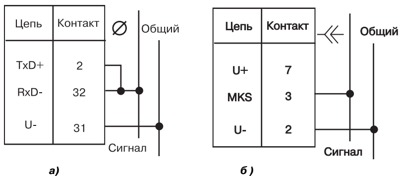
Рисунок В.1 - Схема подключения вычислителей КАРAT-M к сети вычислителей, с помощью:
